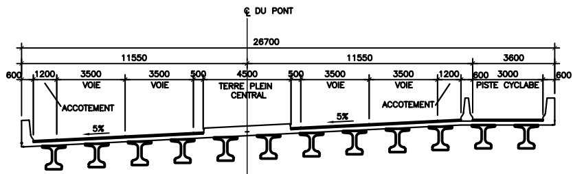
TABLIER AVEC DES POUTRES NETB 1200 COUPE
