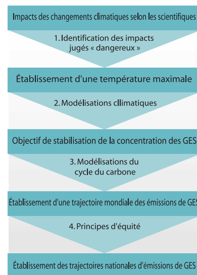
FIGURE 3. Suite logique des étapes à suivre : identification des impacts possibles des changements climatiques (section 2.2), établissement d'une limite de température (section 2.3.1), objectif de concentration des GES dans l'atmosphère (section 2.3.2), objectifs de réduction des émissions à l'échelle mondiale (section 3.1) et nationale (3.2.1)
