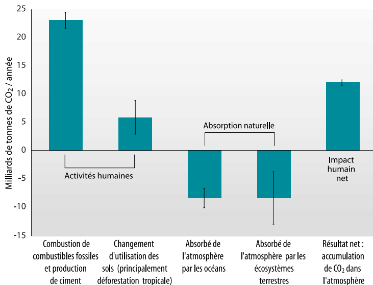
FIGURE 6. Bilan des mouvements de CO 2 dans l'atmosphère de 1989 à 1998. À gauche, le CO 2 ajouté dans l'atmosphère par les activités humaines; au centre, le CO 2 absorbé naturellement par les océans et les écosystèmes terrestres; à droite, l'accumulation nette dans l'atmosphère. Les lignes verticales représentent la plage d'incertitude. 3
