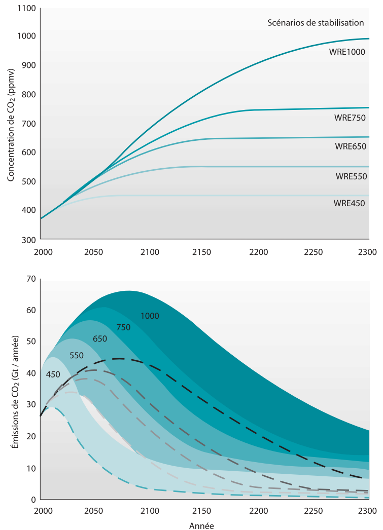
FIGURE 7. Scénarios de stabilisation de la concentration de CO 2 dans l'atmosphère (en haut) et trajectoires des émissions annuelles de CO 2 correspondant à chaque scénario (en bas) avec plage d'incertitude. Les lignes pointillées indiquent la limite inférieure de chaque plage d'incertitude. 5
