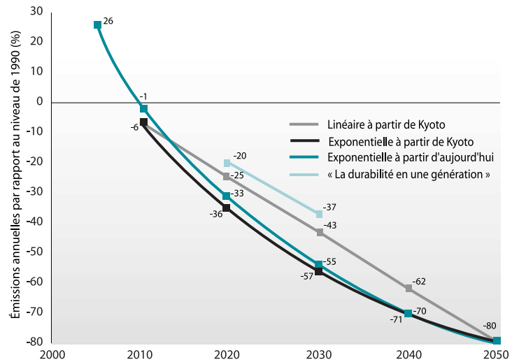
FIGURE 8. Trajectoires possibles pour une réduction radicale des GES émis par le Canada. Nous proposons d'adopter la trajectoire « Linéaire à partir de Kyoto ».
