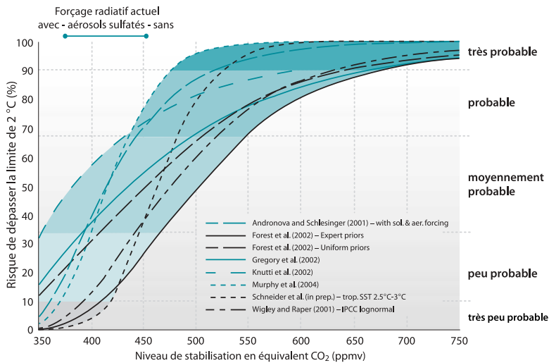
FIGURE 4. Risque d'une augmentation à long terme de plus de 2 °C de la température moyenne à la surface de la Terre par rapport à l'ère préindustrielle, en fonction de différents niveaux de stabilisation de la concentration des GES 64
