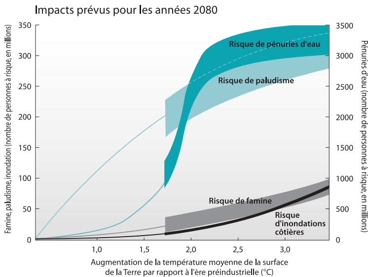
FIGURE 2. Nombre supplémentaire de personnes à risque (en millions) en fonction de différents impacts associés à l'augmentation de la température mondiale 39
