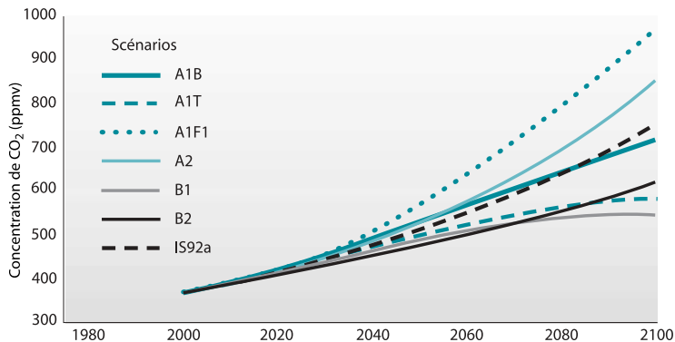
FIGURE 5. Concentrations de CO 2 dans l'atmosphère en l'absence de gestes énergétiques pour limiter les émissions de GES, en fonction des différents scénarios d'émissions du GIEC 78
