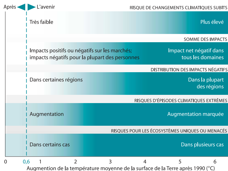
FIGURE 1. Résumé schématisé des impacts prévus par le GIEC en fonction de l'augmentation de la température mondiale 31
