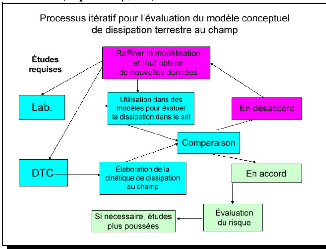
Figure 2 Processus itératif pour l'évaluation des résultats de DTC dans le cas d'un modèle conceptuel spécifique à un pesticide (d'après Purdy, 2002)
