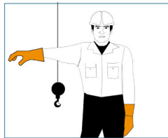
▲ Open clam Ouverture de la benne
