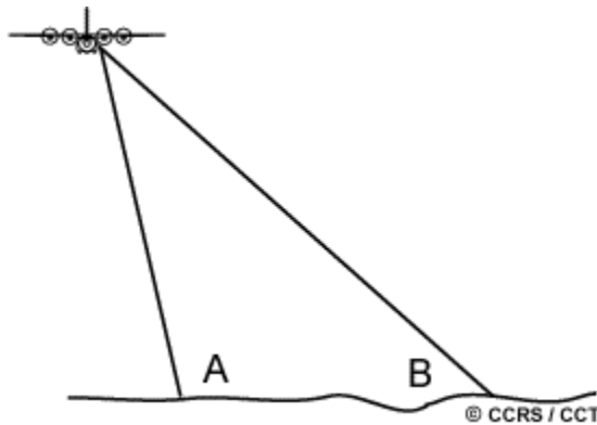
courte portée
