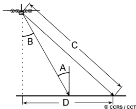
L'angle d'incidence
