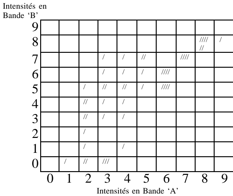
FIGURE 7 Histogramme bidimensionnel.
