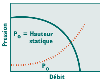
RÉSISTANCE FIXE À PRESSION STATIQUE P \sim (Q^2) + P_o POMPE POUR RÉSERVOIR
