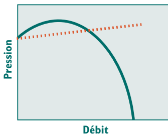
RÉSISTANCE VARIABLE À PRESSION STATIQUE P = \text{CONSTANTE} VENTILATEUR À TIRAGE INDUIT
