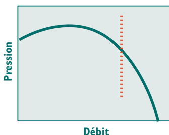
RÉSISTANCE VARIABLE À DÉBIT CONSTANT Q = \text{CONSTANT} TRANSPORTEUR PNEUMATIQUE
