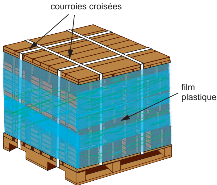
Figure 7 : Emballage à trois épaisseurs de film plastique autour de la palette
