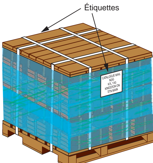
Figure 11 : Apposition des étiquettes sur deux côtés d'une palette ou d'un monoteneur
