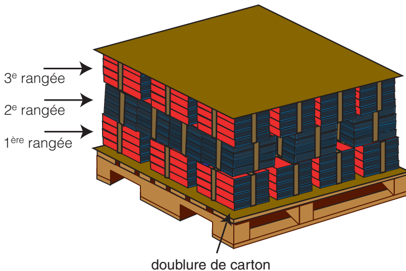
Figure 4 : Palette montrant le placement de la doublure de carton et des liasses
