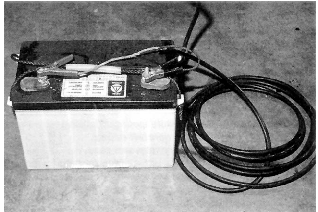
FIGURE 9. 12 Volt Power Hookup.
