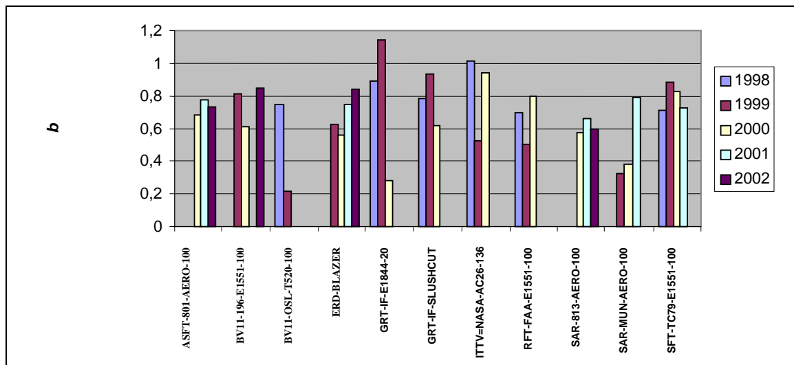
Figure 1 – Multiplicateur b en fonction de l'année (1998-2002) par appareil
