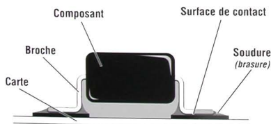
montage en aile de mouette
