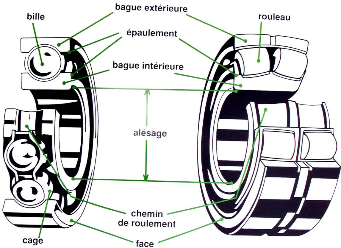
roulement à billes
