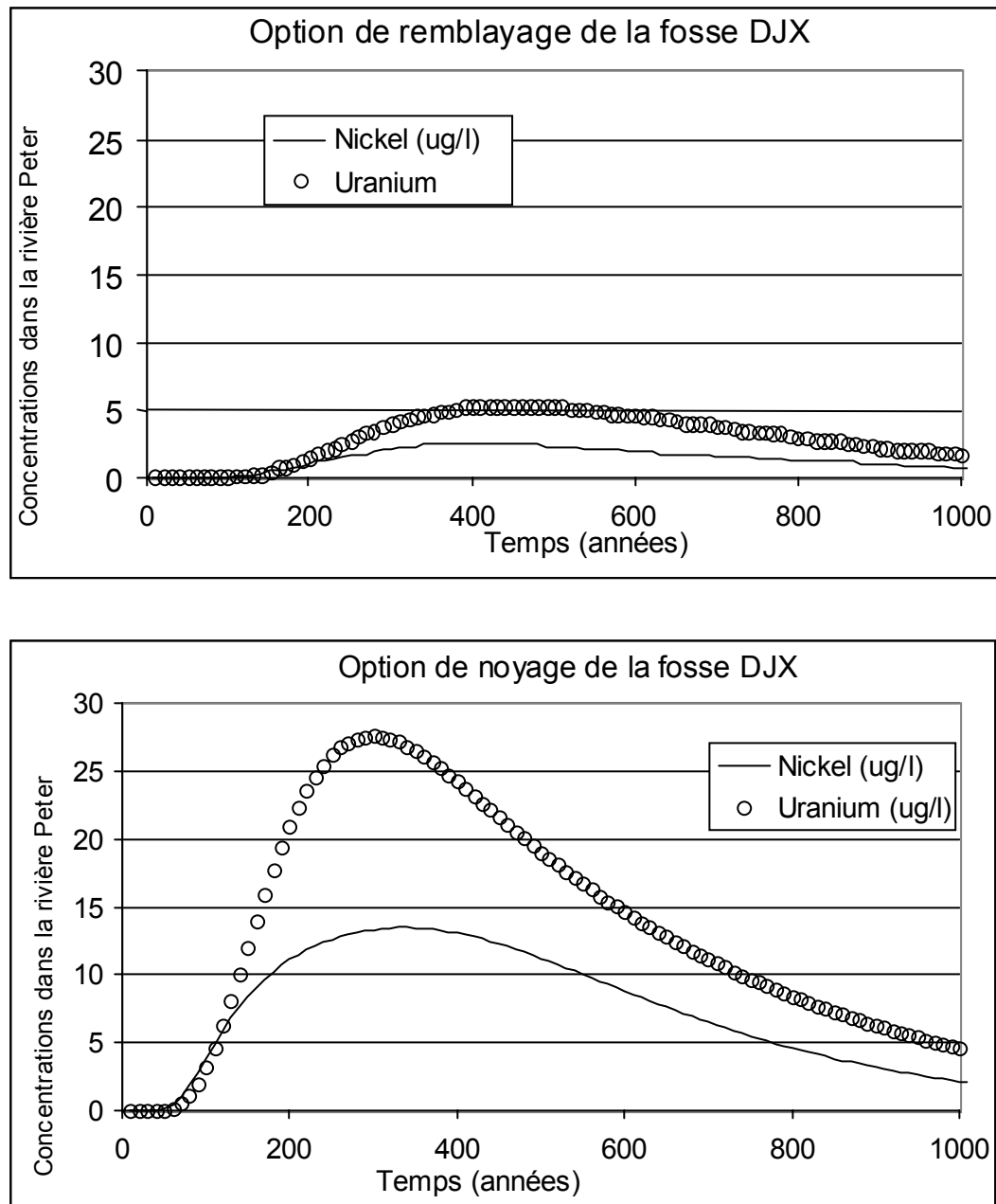
Figure 9.3: Concentrations prédites d'uranium et de nickel dans la rivière Peter pour les scénarios de remblayage et de noyage de la fosse DJX
