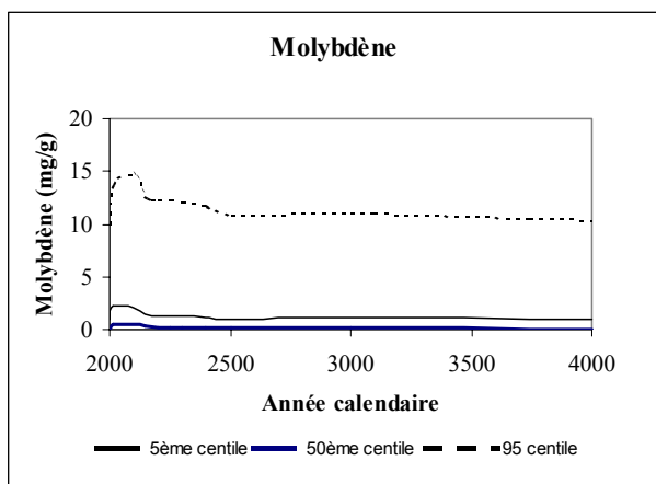
Figure 9.7: Niveaux prédits des contaminants dans les sédiments du lac Cluff au cours des 2000 premières années après le déclassement (suite)
