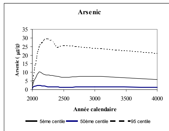
Figure 9.7: Niveaux prédits des contaminants dans les sédiments du lac Cluff au cours des 2000 premières années après le déclassement (suite)
