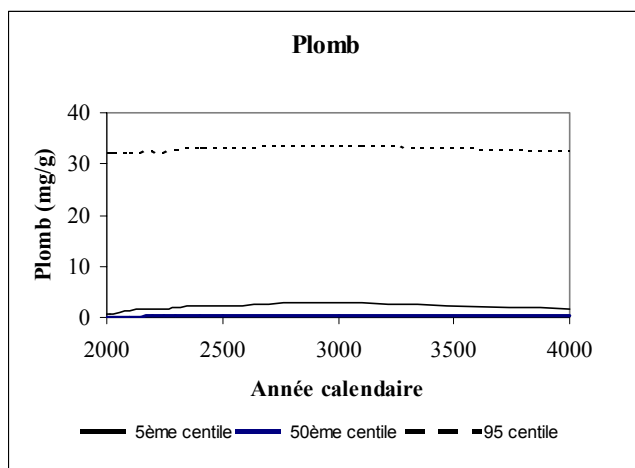
Figure 9.7: Niveaux prédits des contaminants dans les sédiments du lac Cluff au cours des 2000 premières années après le déclassement
