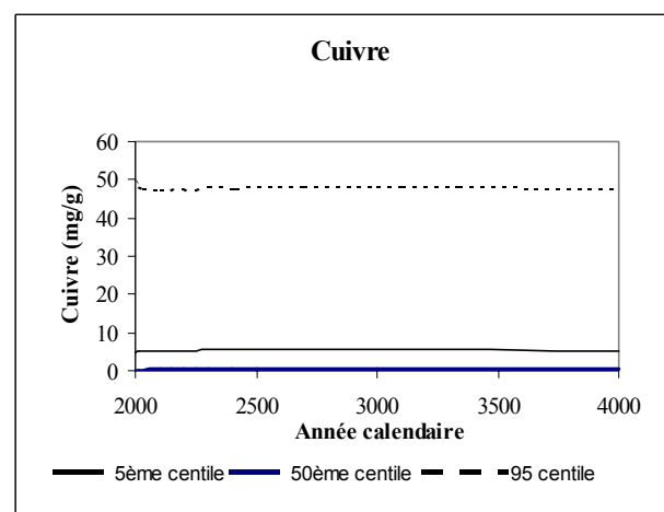
Figure 9.7: Niveaux prédits des contaminants dans les sédiments du lac Cluff au cours des 2000 premières années après le déclassement
