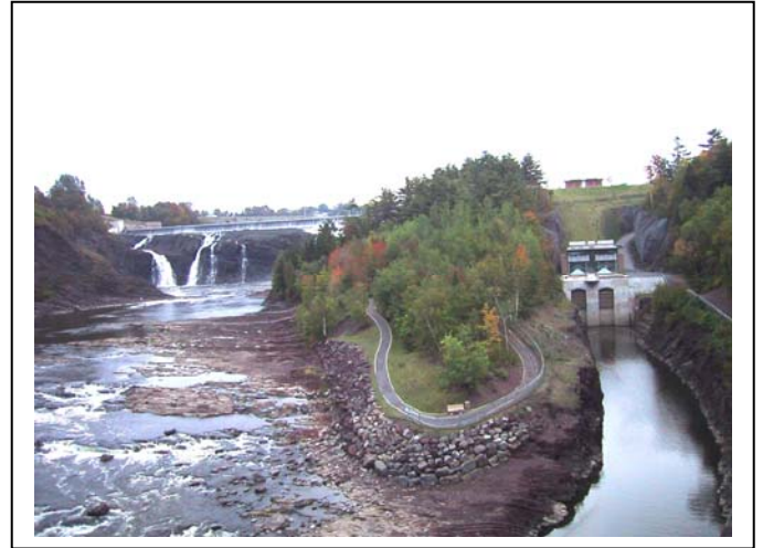
Centrale hydroélectrique du Parc des Chutes-de-la-Chaudière (24 MW), à Lévis (Québec)
