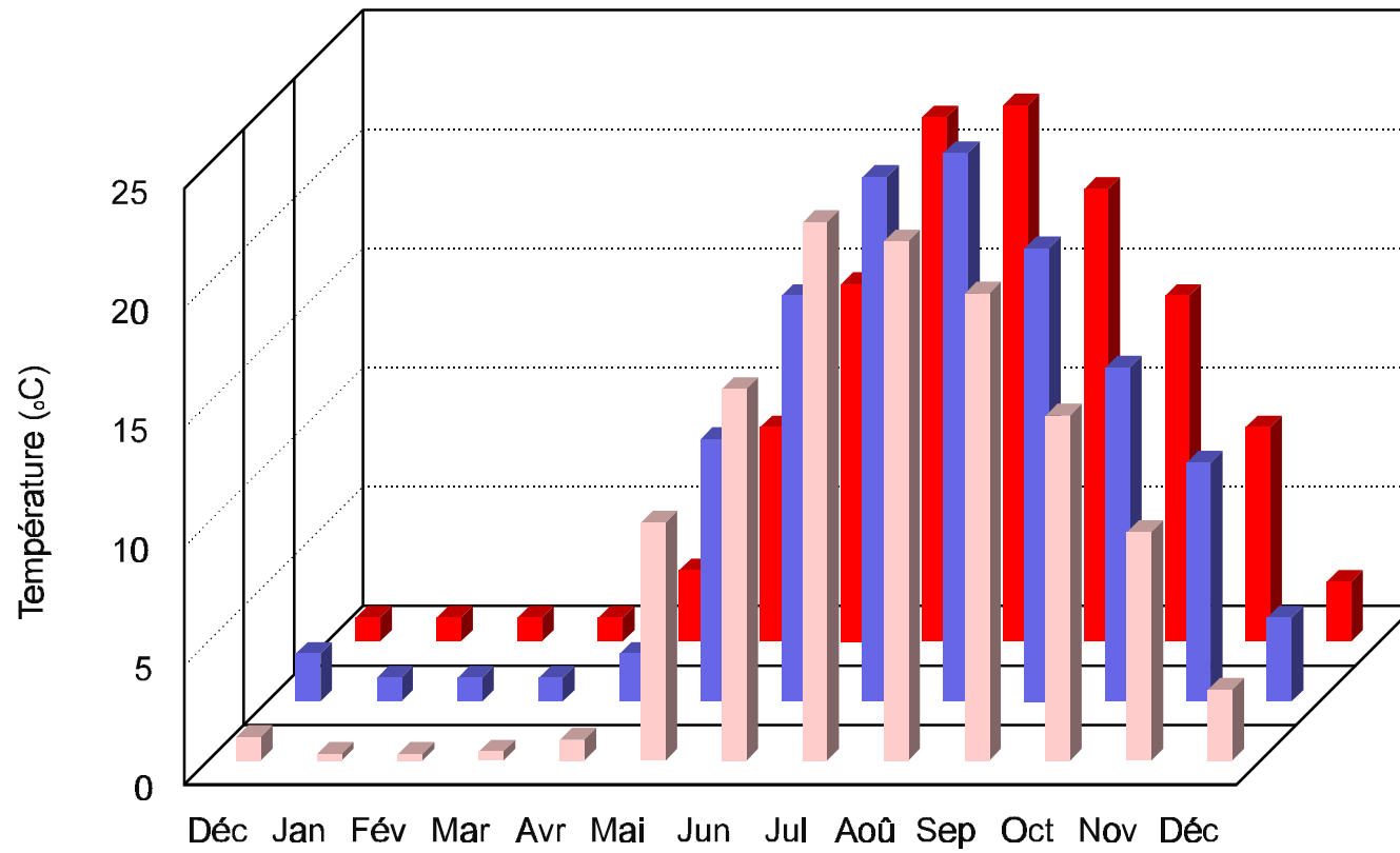
Figure 1. Variation mensuelle de la température (°C) de l'eau pour les usines de traitement d' Ottawa ■ , de Hull ■ , et de Buckingham ■ .
