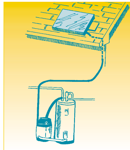
▲ Les installations de petite capacité comprennent un échangeur de chaleur et un réservoir de préchauffage couplés à un chauffe-eau auxiliaire.
