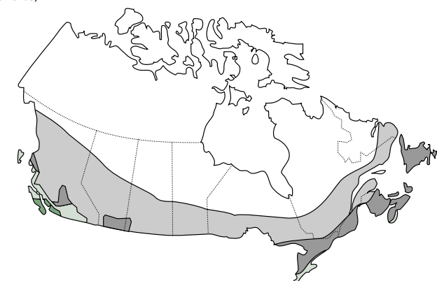
Figure 14 : Coefficient de performance de la saison de chauffage (CPSC) pour les pompes géothermiques à circuit ouvert au Canada (de gauche à droite)
