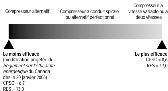
Figure 4 : Rendement d'une thermopompe à air (région V)
