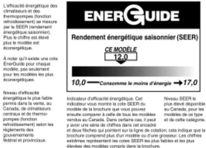
Figure 5 : Cote ÉnerGuide pour les climatiseurs centraux et les thermopompes
