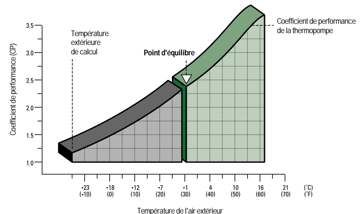
Figure 6 : Particularités du rendement de la thermopompe à air typique
