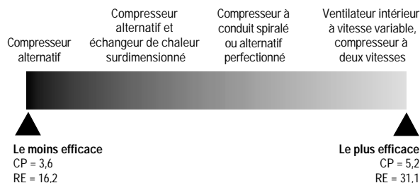
Figure 9 : Rendement des pompes géothermiques à circuit ouvert (température de l'eau à l'entrée de 10 °C)
