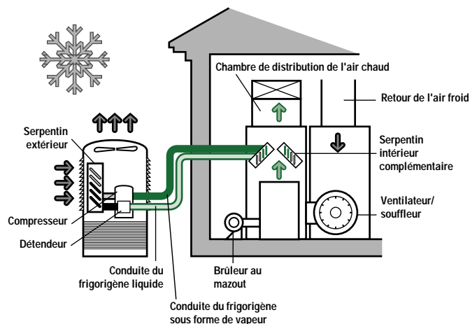
Figure 3 : Thermopompe d'appoint
