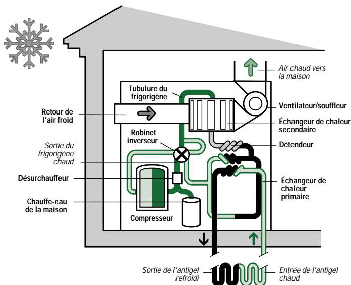
Figure 8 : Éléments de la pompe géothermique typique
