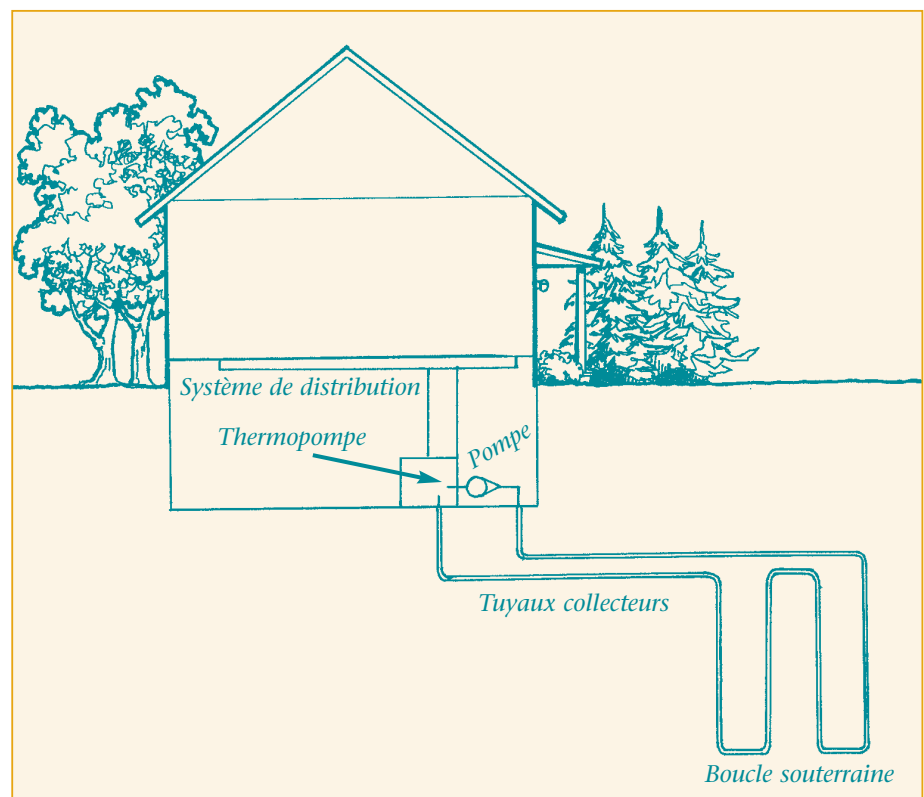
Composants d'un SG ordinaire.
