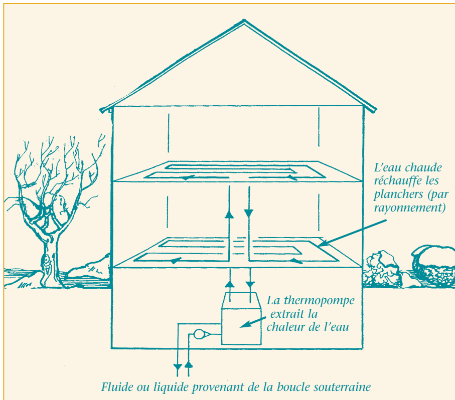
Chauffage à eau chaude dans le plancher.
