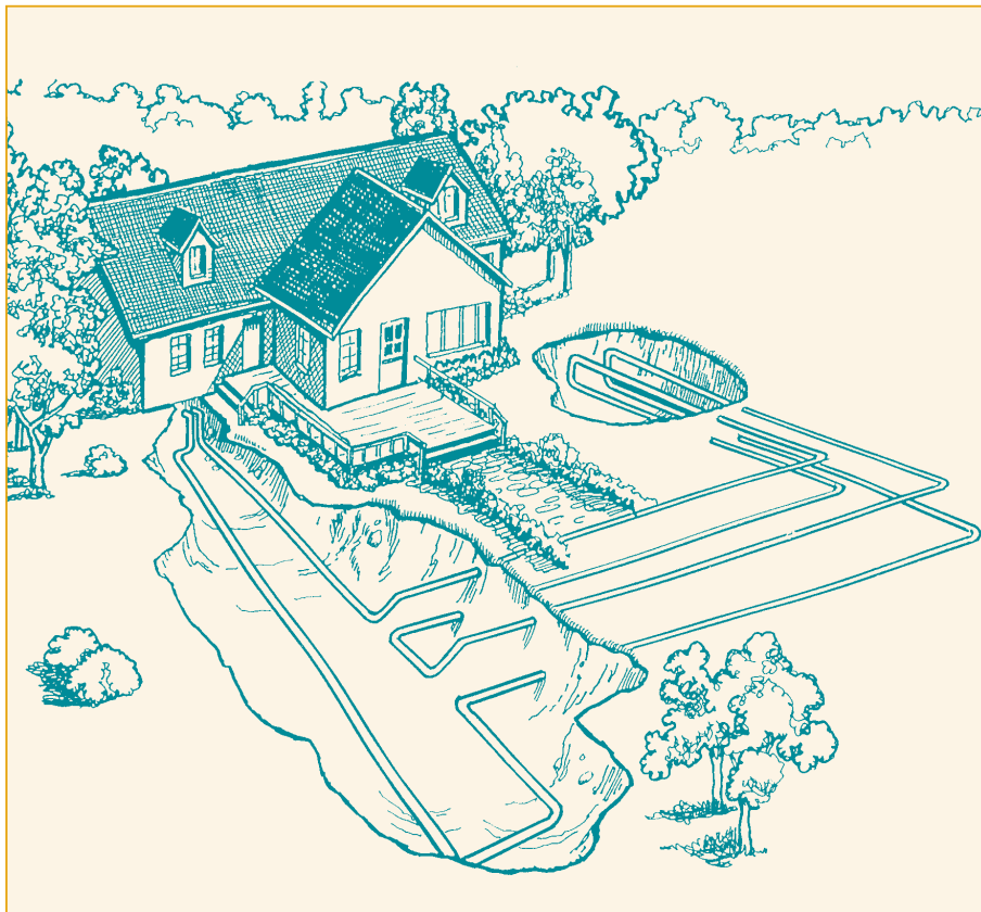
Les boucles souterraines horizontales peuvent chauffer et refroidir votre maison. Elles sont enfouies sous terre.
