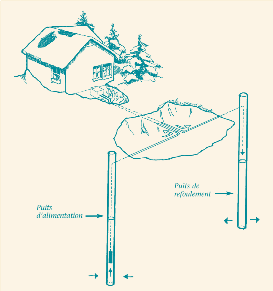
Les systèmes d'eau souterraine, ou circuits ouverts, peuvent chauffer or rafraîchir votre maison, selon vos besoins.
