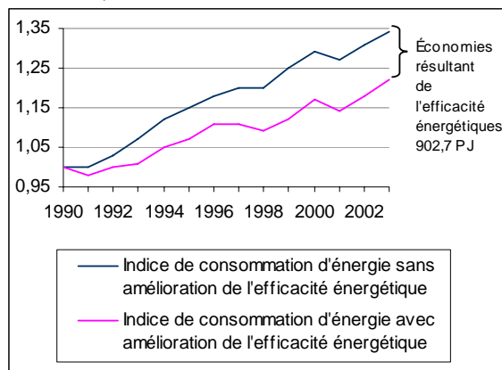
Figure 4.3.1.5 : Consommation d'énergie secondaire, avec et sans amélioration de l'efficacité énergétique, 1990-2004 (Indice : 1990 = 1,0)
