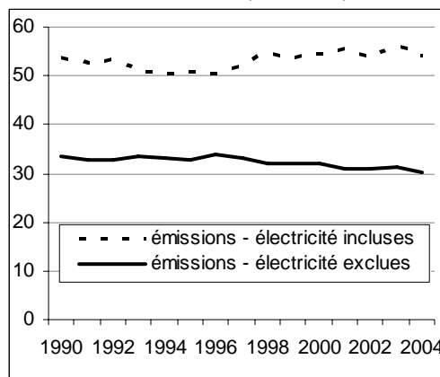
Figure 4.3.2.2 : Intensité en carbone dans le sous-secteur résidentiel (tonne/TJ), de 1990 à 2004
