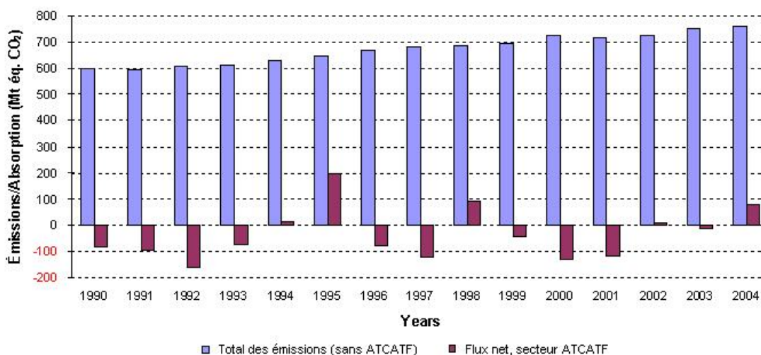
Figure 3.4.6.1 : Flux net dans le secteur ATCATF en comparaison des émissions totales du Canada, de 1990 à 2004
