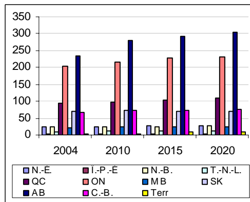
Figure 5.3.10.1 : Émissions de GES par région (Mt d'éq. CO 2 )
