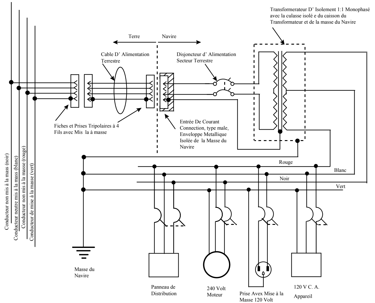
FIGURE 11.1 : Circuit D' Un Transformateur D' Isolement Avec Entrée Monophasé 240 Volts Et Sortie Monophasée 120/240 volts
