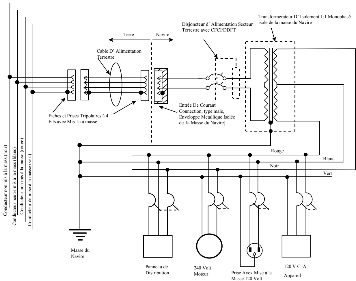
FIGURE 11.2: Circuit D' Un Transformateur D' Isolement Avec Entrée Monophasée 240 Volts Et Sortie Monophasée 120/240 volts Avec La Protection D' Un Disjoncteur Differential (GFCI/DDFT) Au Primaire Du Transformateur
